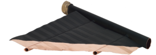
SUNSHINE BCC SERİSİ (Bakır Siyah Boyalı) SOLAR TERMAL KOLLEKTÖR ABSORBER
